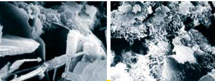
常规砂浆 (左) 与使用Krytol的砂浆 (右)
